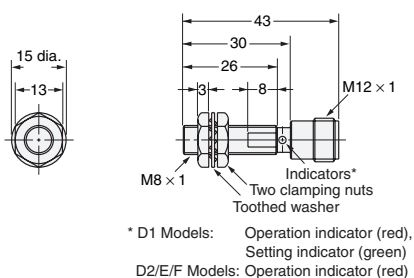
Diagram 18 E2E-X2D□-M1(G) E2E-X1R5E□-M1/E2E-X1R5F□-M1
